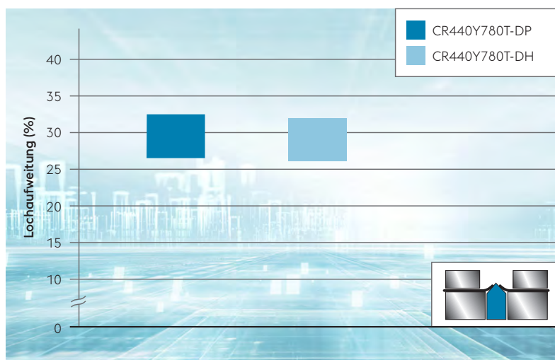
Lochaufweitungversuch nach ISO 16630, typische Werte
