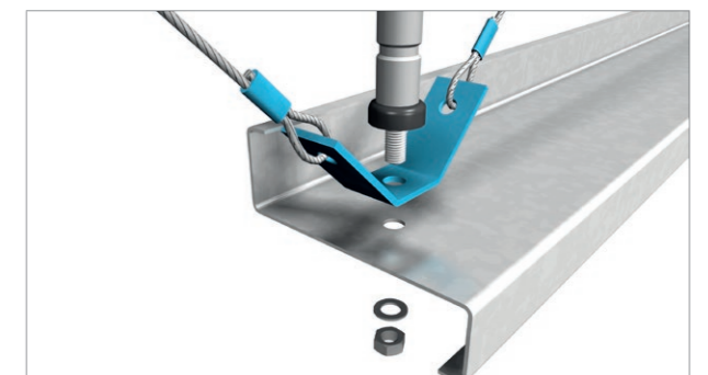
Montagedetail + SadeF-Lock® + doppelte Diagonalabhängung
