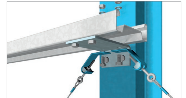
Montagedetail Wandriegel + Wandriegelhalter + Diagonalabhängung
