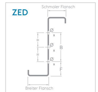
Querschnittswerte: siehe S.105
