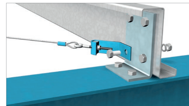
Montagedetail Dachpfette + Pfettenhalter + Diagonalabhängung
