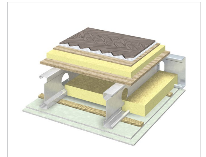
Bühne mit einem schwimmenden Aufbau und hoher Schalldämmung für den Fall einer Geschosdecke in Leichtbauweise.
