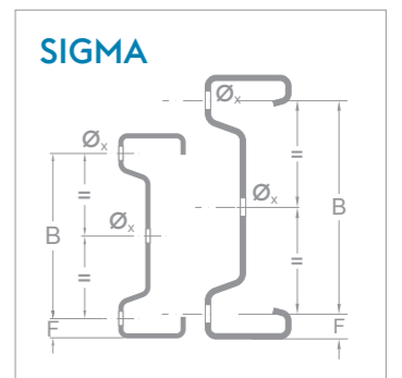
Querschnittswerte: siehe S.102 - 103 - 104
