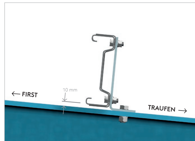
+/- 10 mm Abstand zwischen voestalpine Sadef SIGMA - Querschnitt und Unterkonstruktion.
