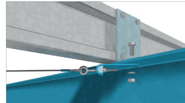
Die Diagonalabhängung wird direkt am Binder befestigt, indem die vorhandenen Lochungen für die Pfettenhalter genutzt werden. Die Montage erfordert so kein zeitaufwendiges Bohren von zusätzlichen Löchern.**
