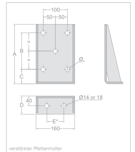
verstärkter Pfettenhalter Symmetrische Lochungen im unteren Teil des Pfettenhalters für abweichende Lochbilder bitte voestalpine Sadef kontaktieren. E*: dieses Mass kann zwischen 50 bis 100 mm variieren (standard 70 mm, Ø 18)
