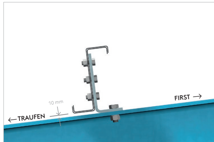
+/- 10 mm Abstand zwischen voestalpine Sadef ZED-Querschnitt und Unterkonstruktion.
