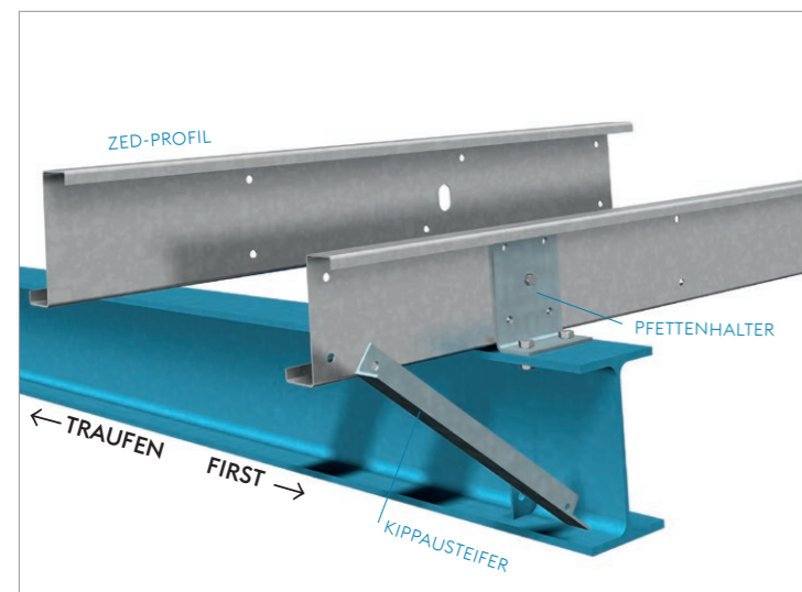
+/- 10 mm Abstand zwischen voestalpine Sadef ZED-Querschnitt und Unterkonstruktion.
