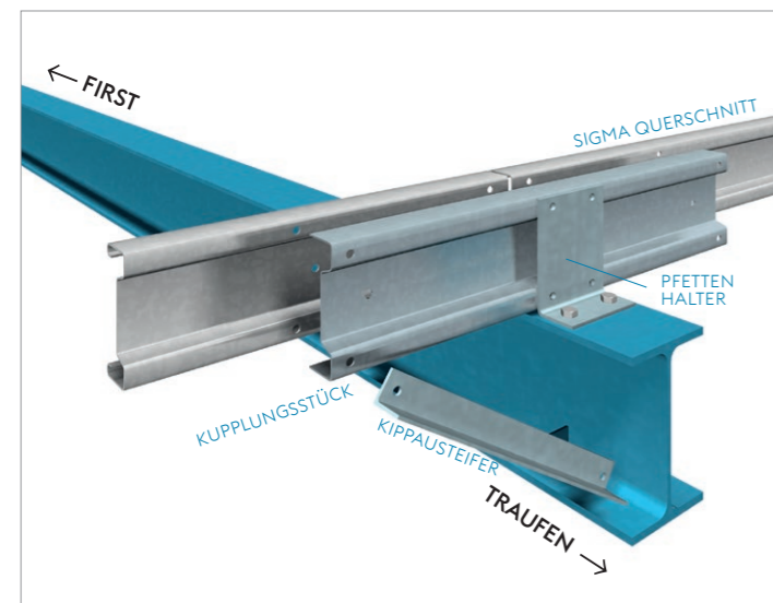
+/- 10 mm Abstand zwischen voestalpine Sadef SIGMA - Querschnitt und Unterkonstruktion.
