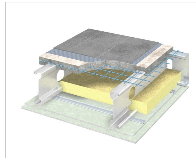
Bühne mit integriertem Betonboden (siehe S.78).
