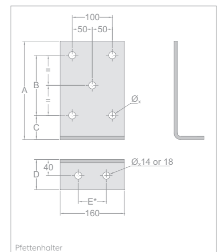
Pfettenhalter Symmetrische Lochungen im unteren Teil des Pfettenhalters für abweichende Lochbilder bitte voestalpine Sadef kontaktieren. E*: dieses Mass kann zwischen 50 bis 100 mm variieren (standard 70 mm, Ø 18)
