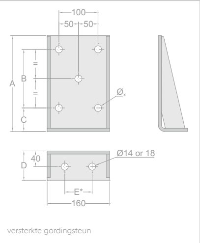
De perforaties worden centrisc in de voet van de gordingsteun aangebracht. Voor afwijkende gatenperforaties: Contacteer voestalpine Sadef. E*: de maat E is vrij te kiezen van 50 tot 100 mm (standaard 70 mm, Ø 18).
