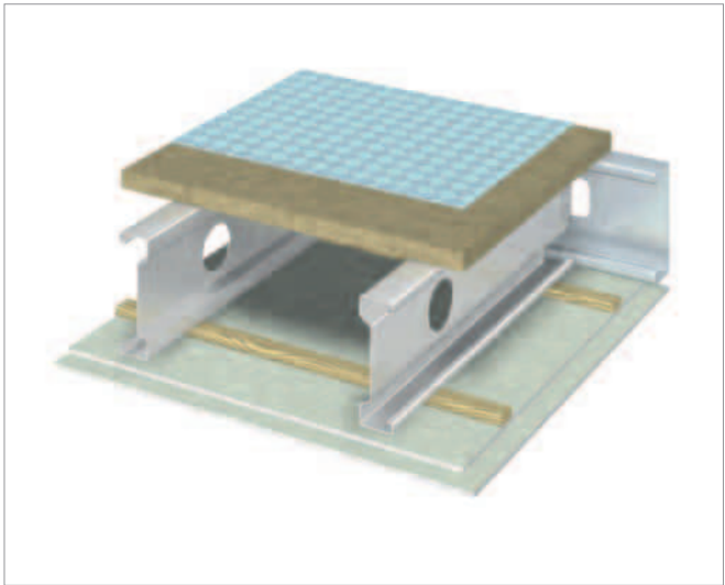
Vloerafwerking met houtvezelplaat met hoge densiteit, eventueel voorzien van een plafondaafwerking ten behoeve van brandweerstand.
