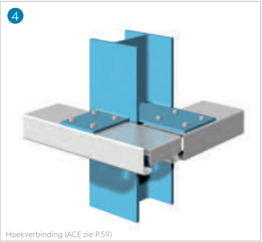
Hoekverbinding (ACE zie P.59)
