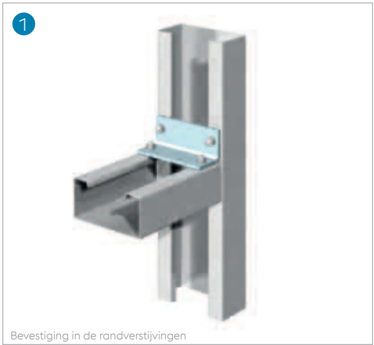
Bevestiging in de randverstijvingen
