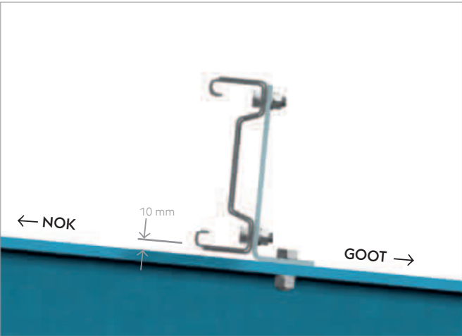
+/- 10 mm speling tussen de voestalpine Sadef SIGMA-profielen en de onderconstructie
