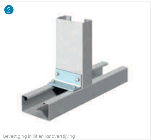
Bevestiging in lijf en randverstijving
