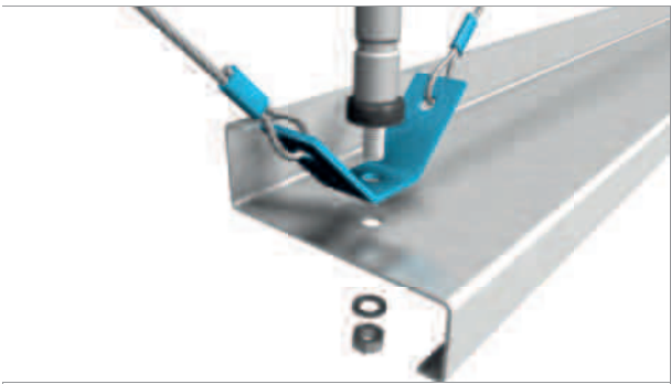
Montagedetail wandregel + Sadef-Lock® + dubbele bretel.
