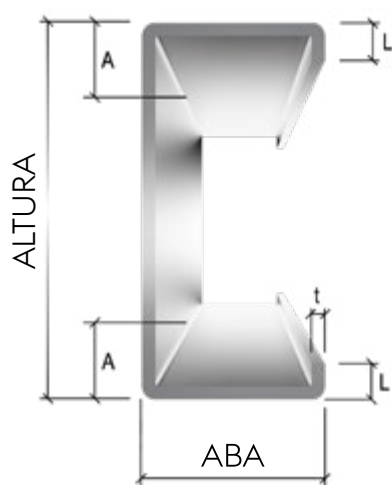
Seção transversal das vigas de mezaninos.
