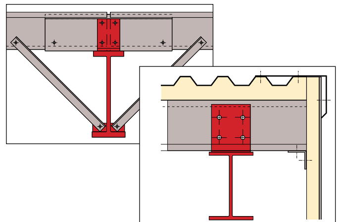
Exemplos de demais componentes do Sistema METSEC.
