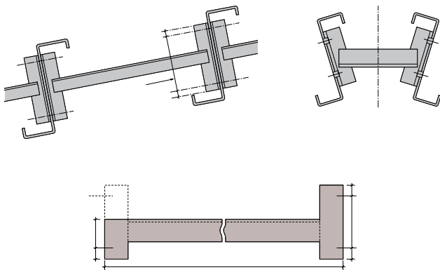
Esquema das correntes ASB, AA e SRS.
