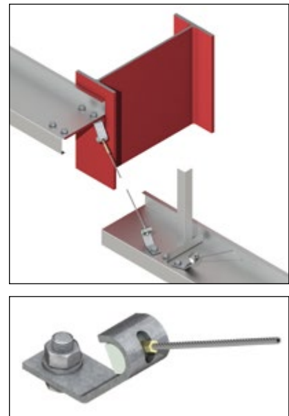
Esquema de tirantes WDT.
