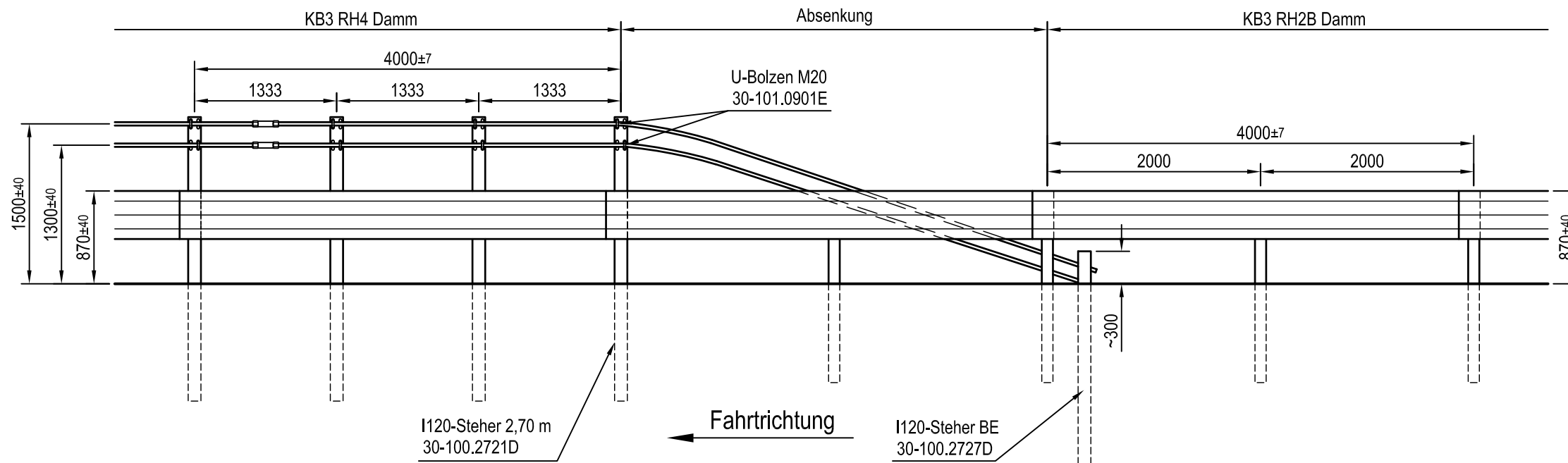
ANSICHT VON VORNE
