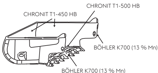
BÖHLER K700 (13 % Mn)
