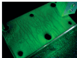
Detección de fisuras mediante partículas magnéticas fluorescentes
