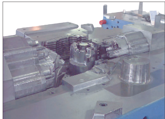
Molde de fundición inyectada de aluminio para la industria automotriz.
