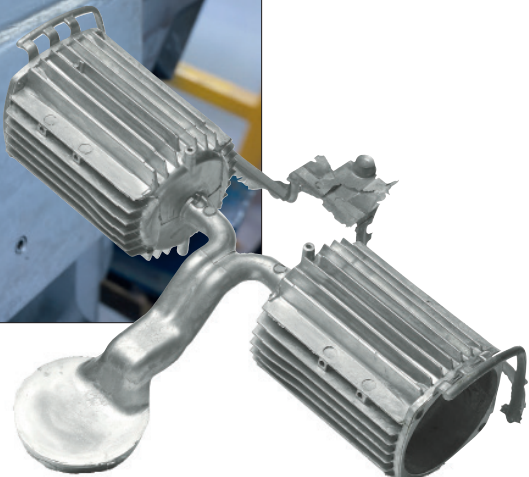
Bomba de aluminio fijado al sistema de llenado, por ejemplo cámaras, puntos de inyección y rebosadero.
