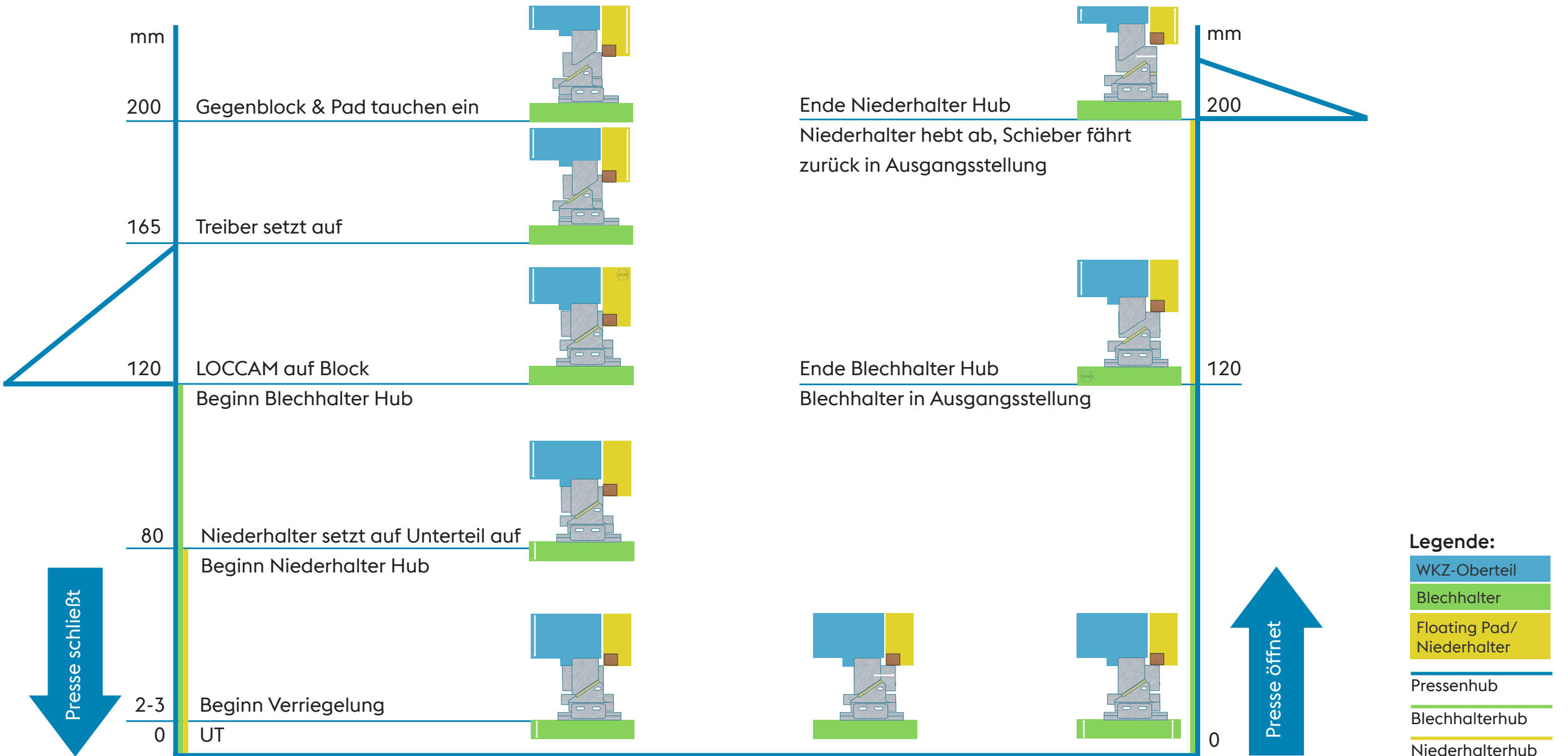
Blechhalter mit LOCCAM gegen Niederhalter verriegelt
