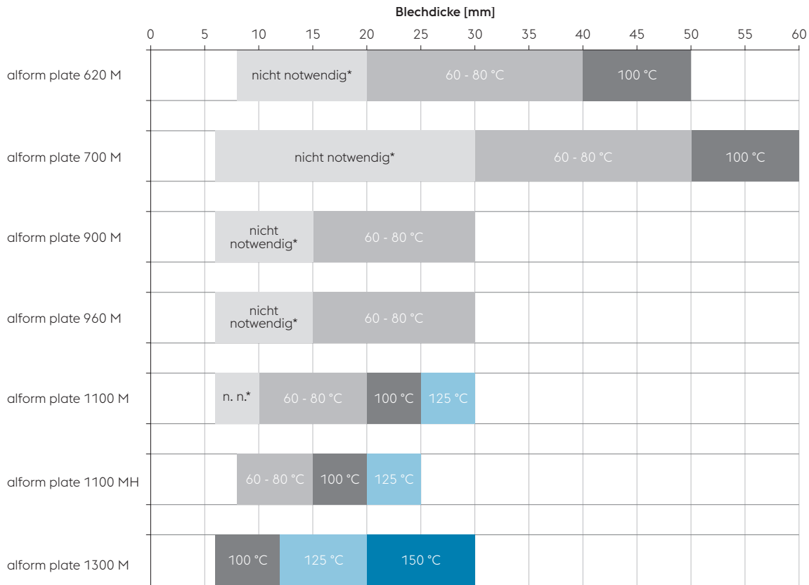
Abbildung 4: Empfohlene Vorwärmtemperaturen beim Schweißen
