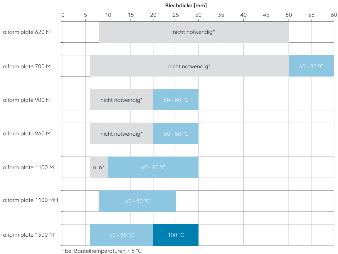
Abbildung 2: Empfohlene Vorwärmtem- peraturen beim thermischen Schneiden
