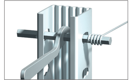
Végezze el a feszítést a leova® End combi feszítőkulccsal. Kész.
