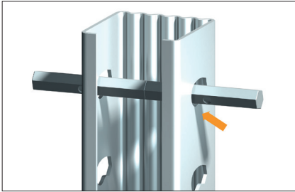
Helyezze be a leova® Sekaduo huzalcsevélőt.
