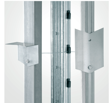
Ankerplatte Endpfahl, Krallenschutz, Ankerplatte Spalierpfahl
