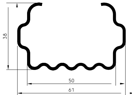
Huzalszélesség: 53 mm
